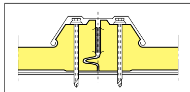
DETALLE DE LA UNIÓN
